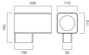
PH11R
